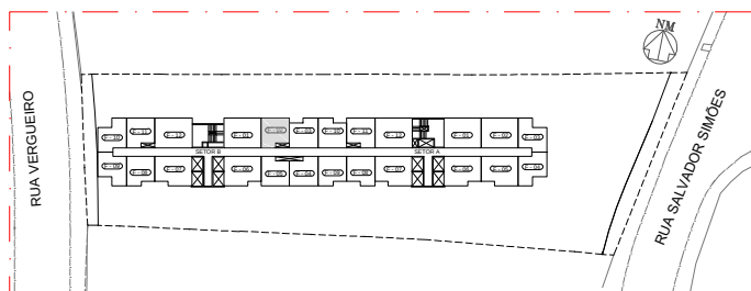
PLANTA LOCALIZAÇÃO - TORRE - PAV. TIPO
